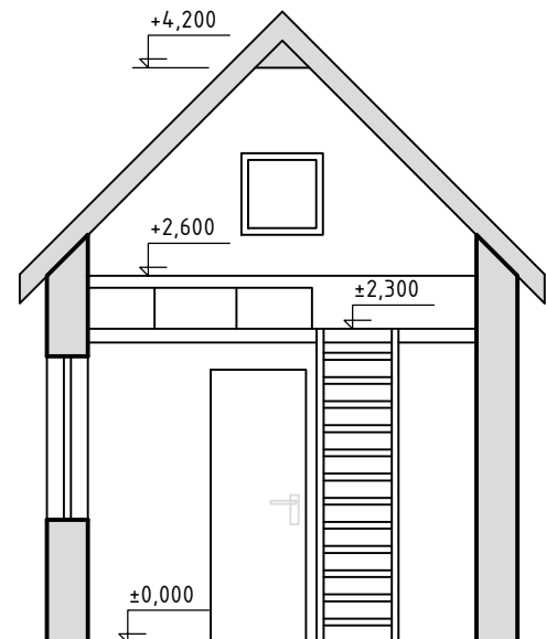
ŘEZ A-A
